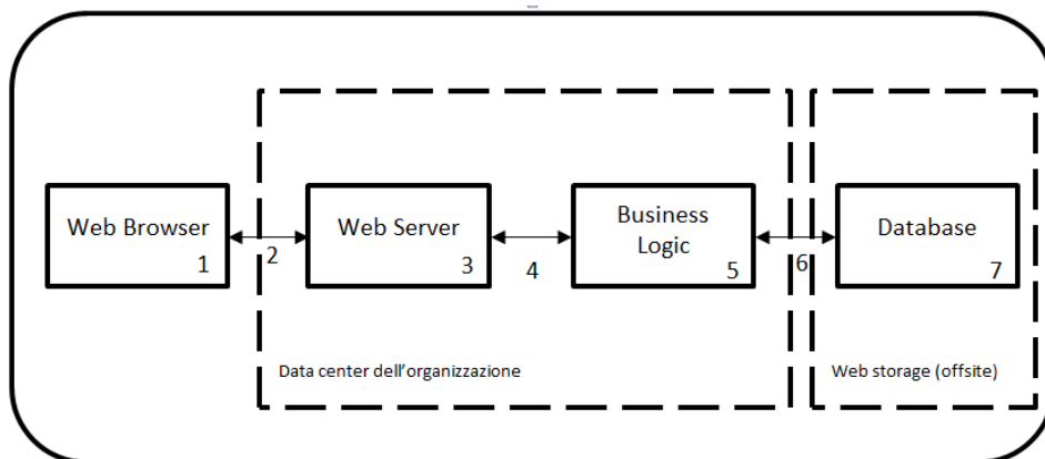
Figura 7 - Numerazione degli elementi del diagramma
